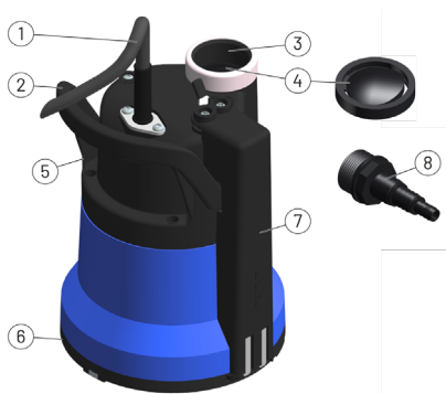
带液位开关的 Simer 6S
