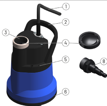
Simer 6 utan nivåbrytare
